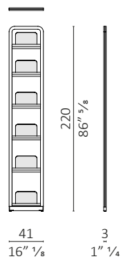
Young Holden fianco di connessione/ connection element
