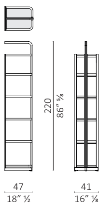
Young Holden modulo terminale stondato/rounded end element
