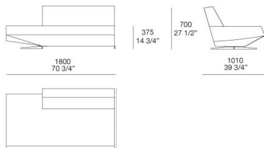
SYPX180 SYPZ180
