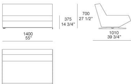
SYCE140
